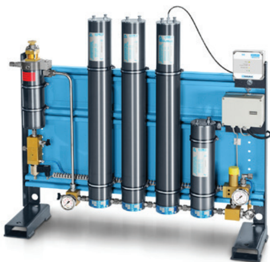
Внешняя фильтровальная система с патроном
